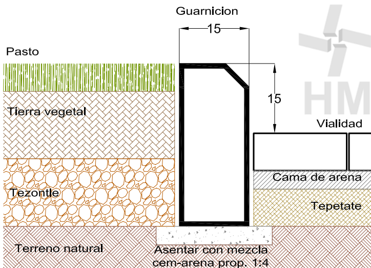
CORTE INSTALACION DE GUARNICION EN CAMELONES Delimitando áreas verdes
