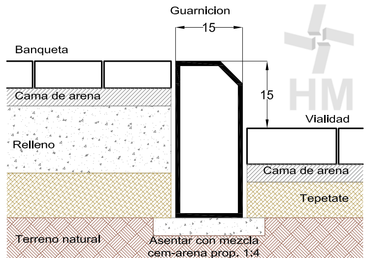
CORTE INSTALACION DE GUARNICION EN BANQUETA Delimitando áreas peatonales
